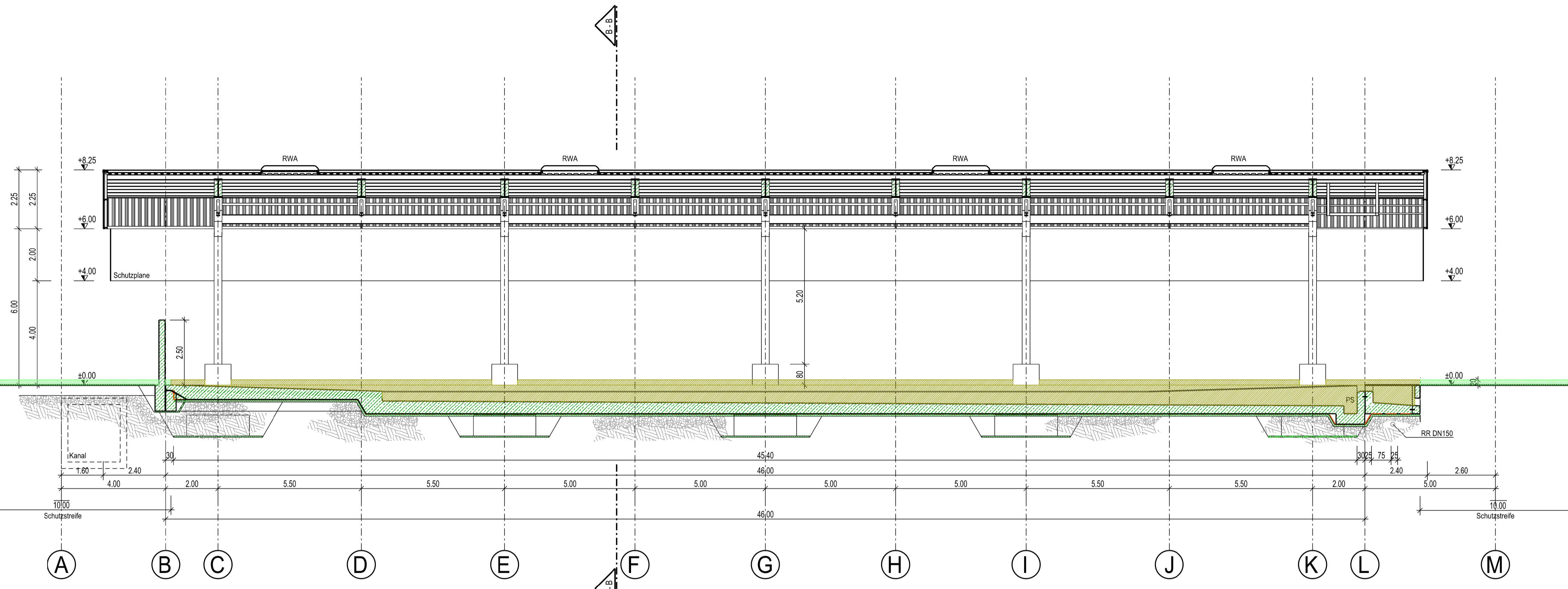
Schnitt A-A
